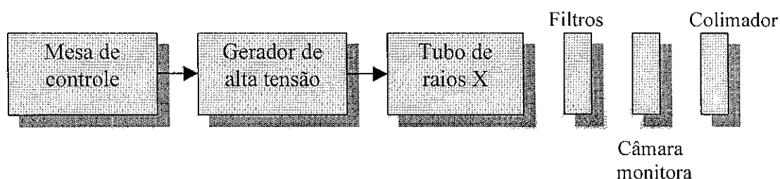
FIG. 3.5 Diagrama em blocos simplificado do gerador de raios X da Siemens, modelo Stabilipan 300.
