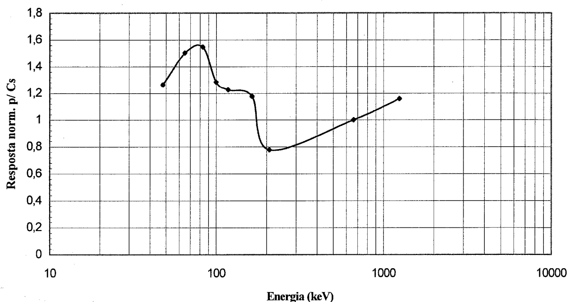
FIG. 4.4 Resposta energética para H*(10), normalizada para o ^{137}\text{Cs} , do MIR 7026 com o detector GM interno com filtro de compensação de alumínio e chumbo com furos concêntricos.
